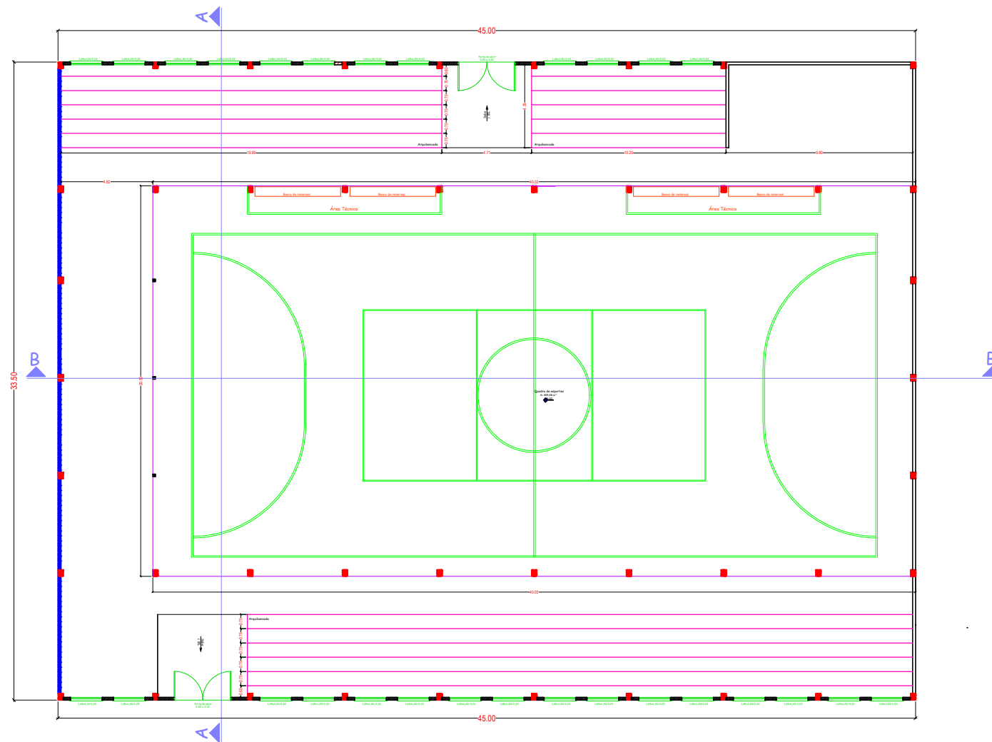
PLANTA BAIXA
